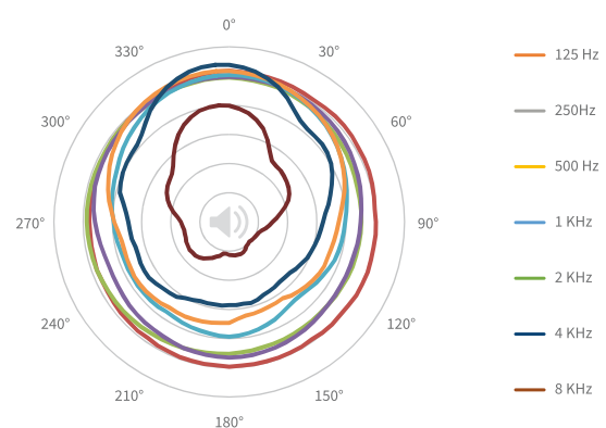
Direttività 1/1 OCT
